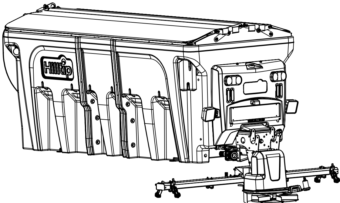
IceStriker™ 1250 AML
